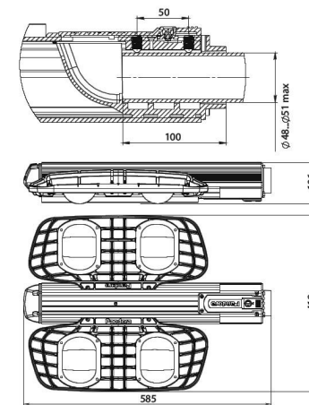
Рисунок 3. Габаритный чертеж
